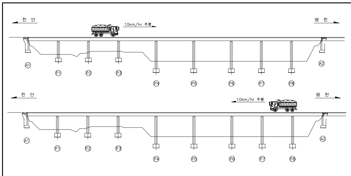
<그림 5.6> 의사정적 주행방향(양방향)
