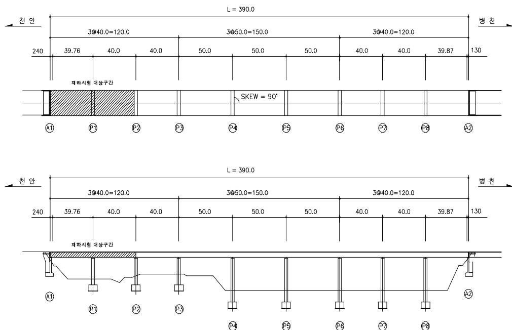
<그림 5.4> 재하시험 대상경간
